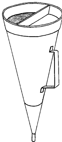
Figura 2. Viscosímetro Marsh.
